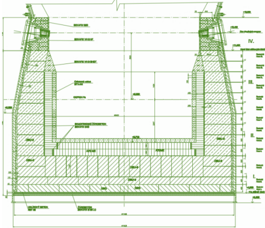
VÝZDÍVKA NÍSTĚJE VP3
